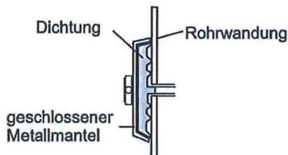
Beispiel Spannverbinder
