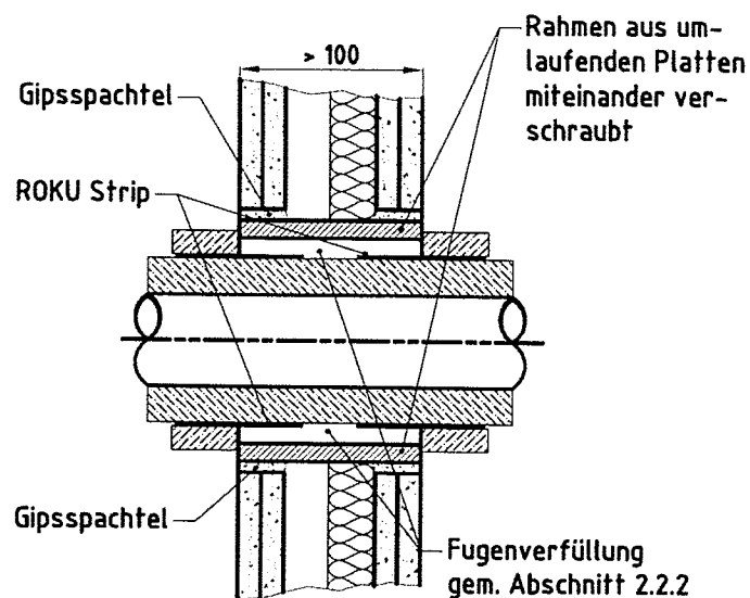
Einbau von Rahmen (Platten verschraubt)
