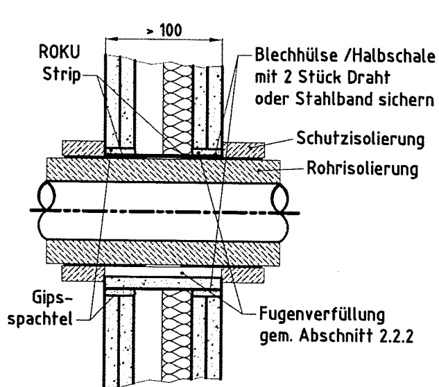
Einbau von Blehhülsen oder Halbschalen
