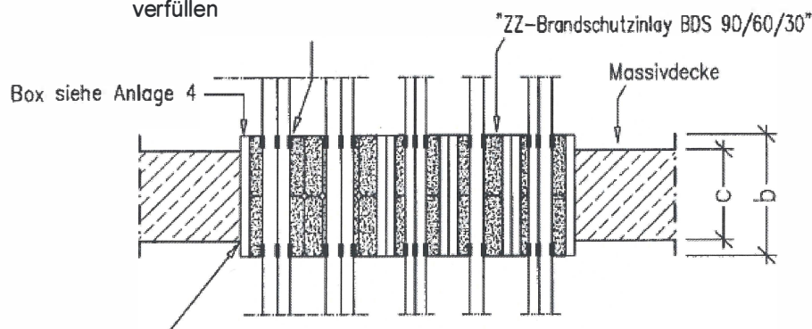
Schnitt A-A
